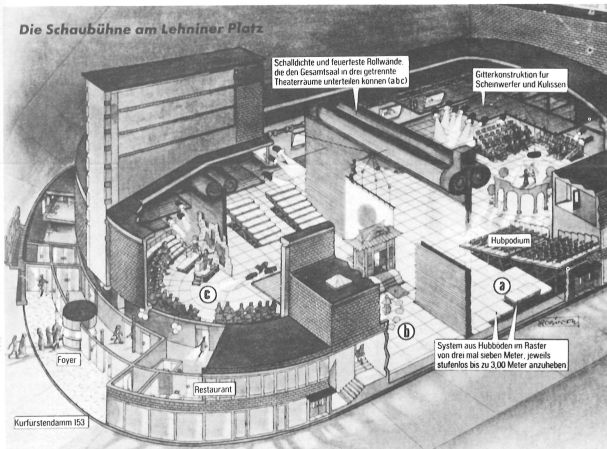
Schaubühne — dwarsdoorsnede
